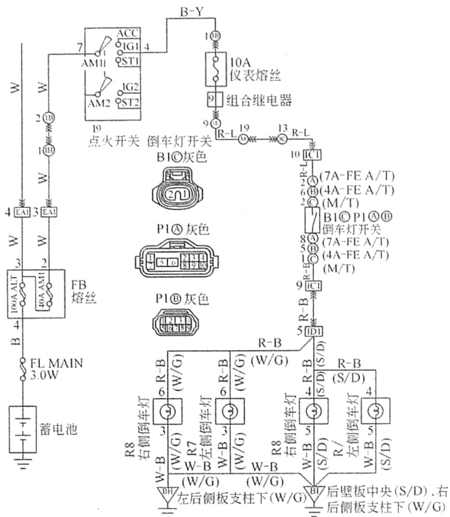
图 22-3-1 倒车灯电路图
